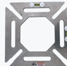
Crosse tourne poteau Type D REF : 24 - 0001 (l : 1m90) REF : 24 - 0002 (l : 1m)
